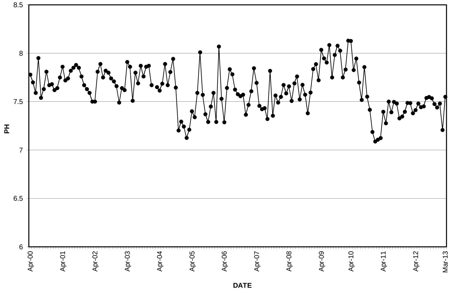
GRAPH 41 pH MIDDLE QUINSAM LAKE INLET (WA)
