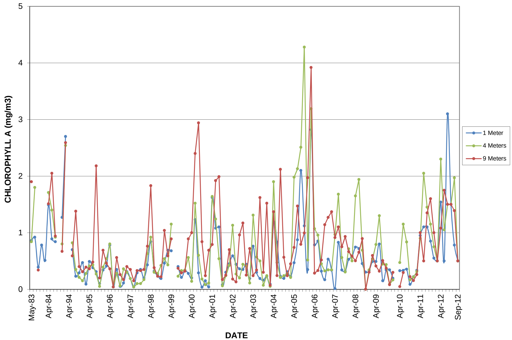
GRAPH 50 LONG LAKE CHLOROPHYLL A
