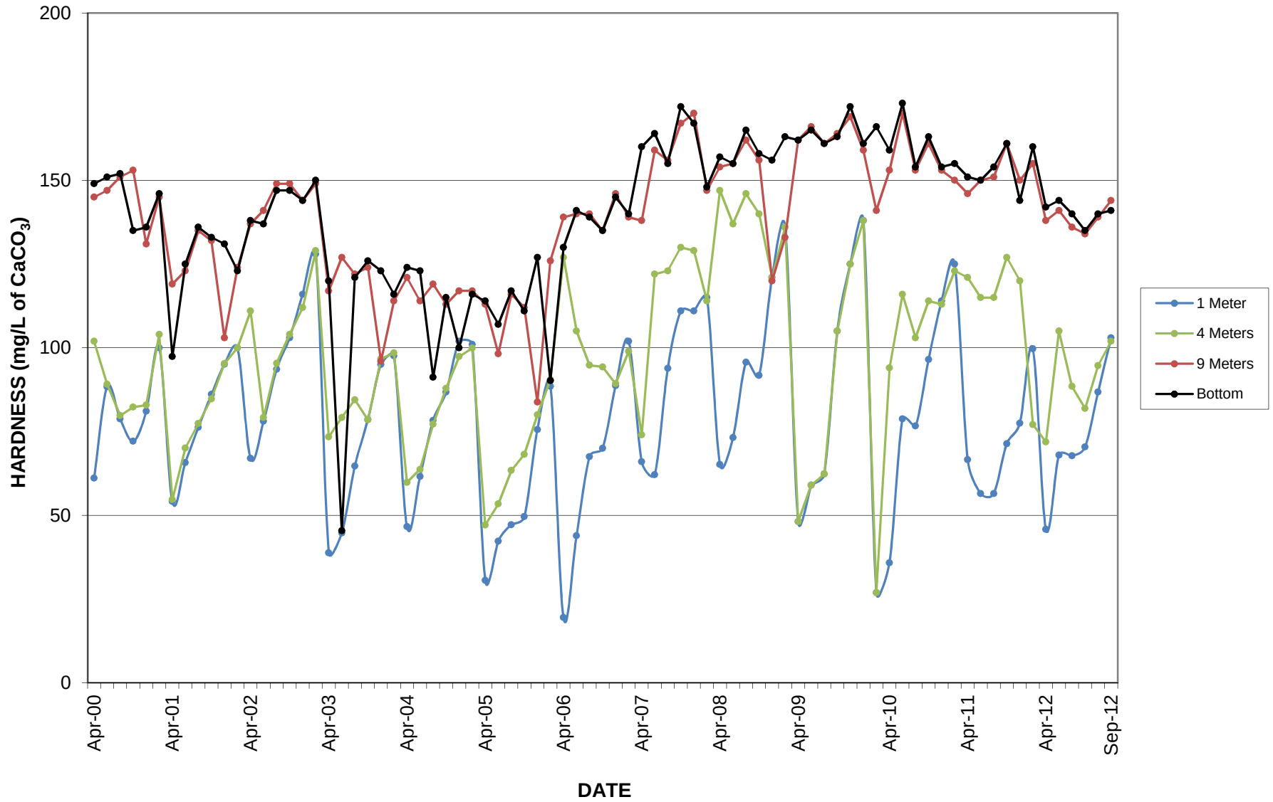
GRAPH 47 LONG LAKE HARDNESS
